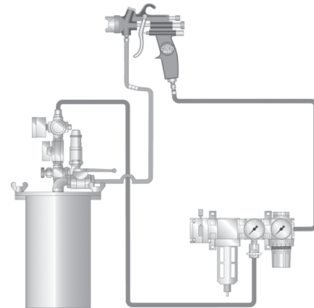
Anschlussschema für Materialanschluss
